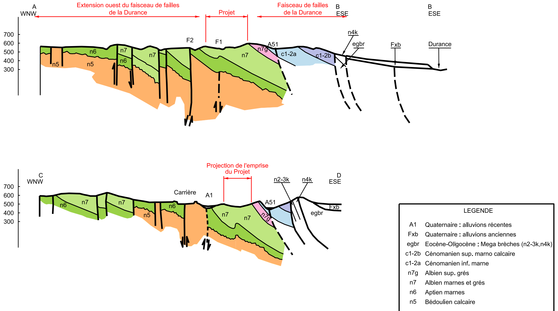
Figure 3.4 : Coupes géologiques interprétatives 1 / 25 000
